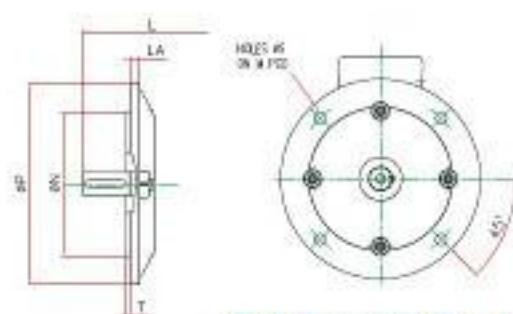
FLANGE MOUNTING IM - B5
