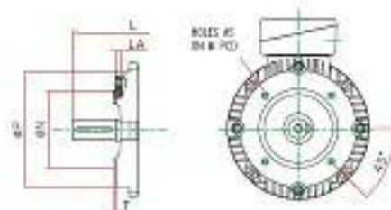
FACE MOUNTING IM - B14
